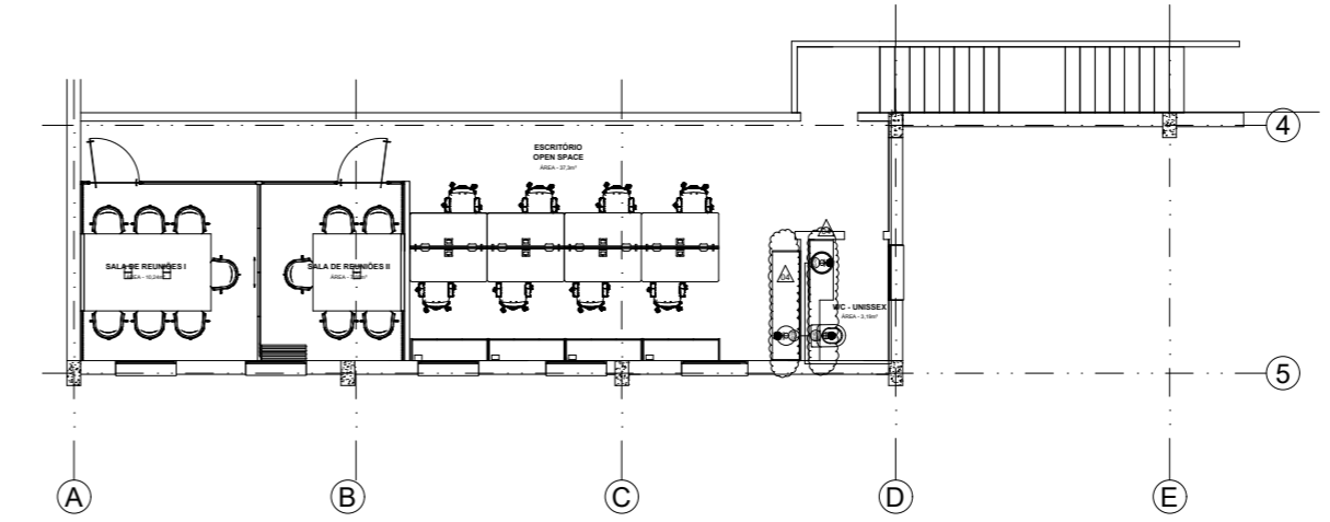
PLANTA BAIXA - 1º PAVIMENTO - ESCRITÓRIO Hidráulica - Pontos de Água
