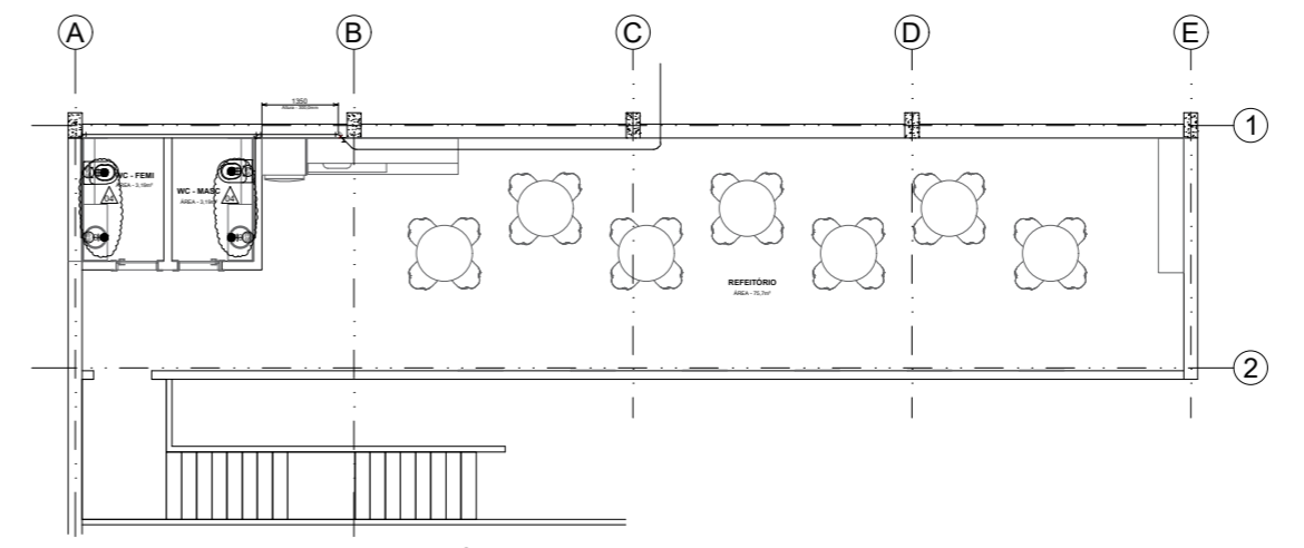
PLANTA BAIXA - 1º PAVIMENTO - REFEITÓRIO Hidráulica - Pontos de Água
