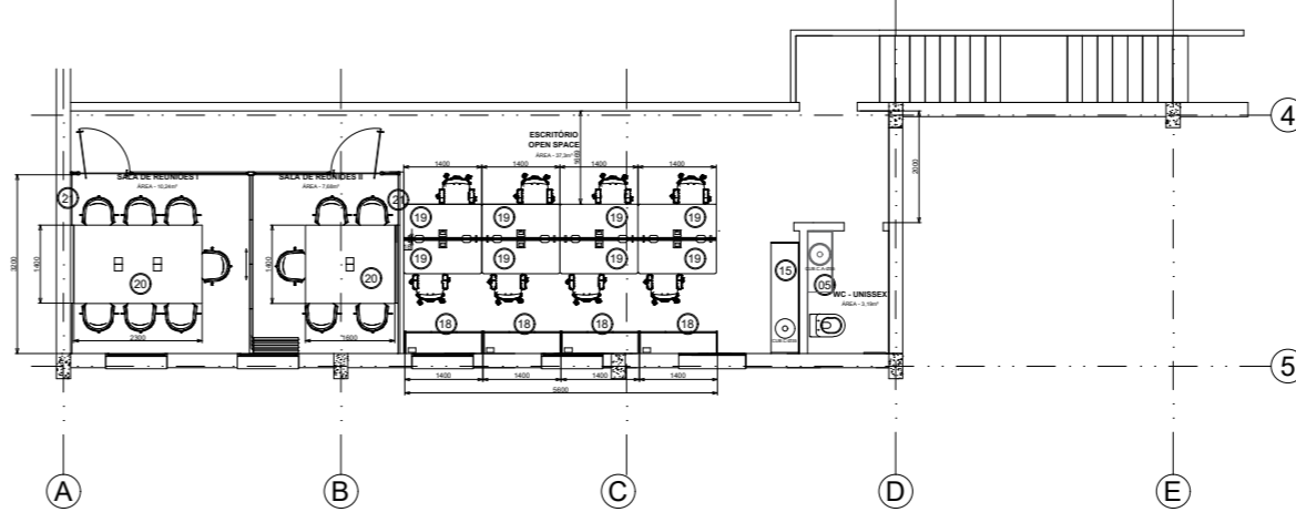
PLANTA BAIXA - 1º PAVIMENTO - ESCRITÓRIO Layout Mobiliário
