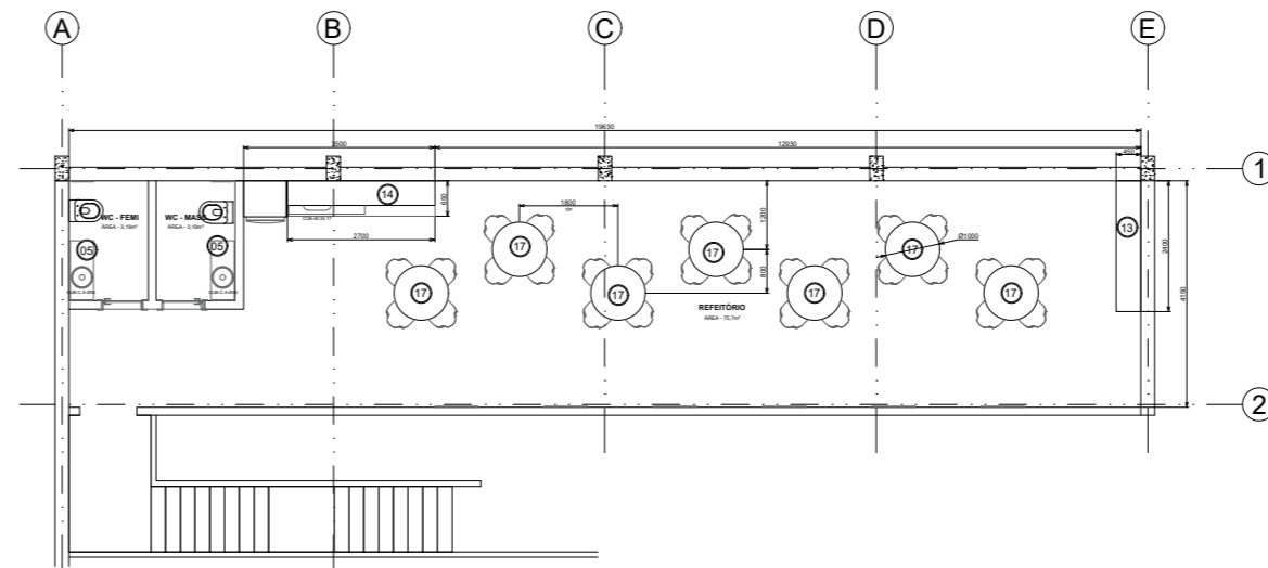
PLANTA BAIXA - 1º PAVIMENTO - REFEITÓRIO Layout Mobiliário
