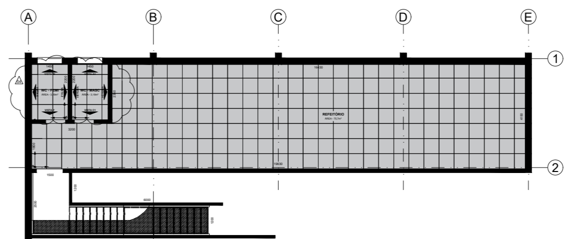
PLANTA BAIXA - 1º PAVIMENTO - REFEITÓRIO Pisos e Revestimentos
